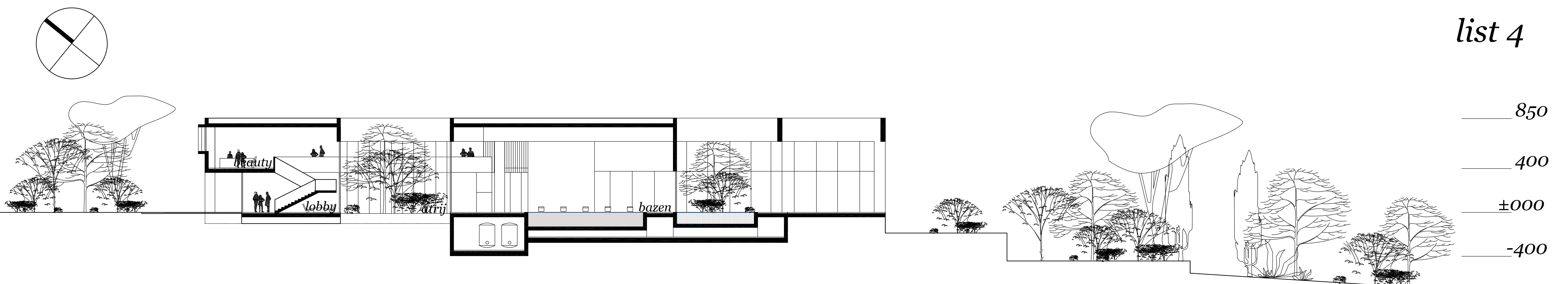
presjek c-c
