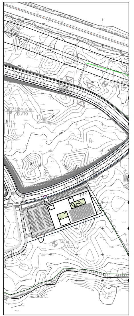
SITUACIJA 1/2000
